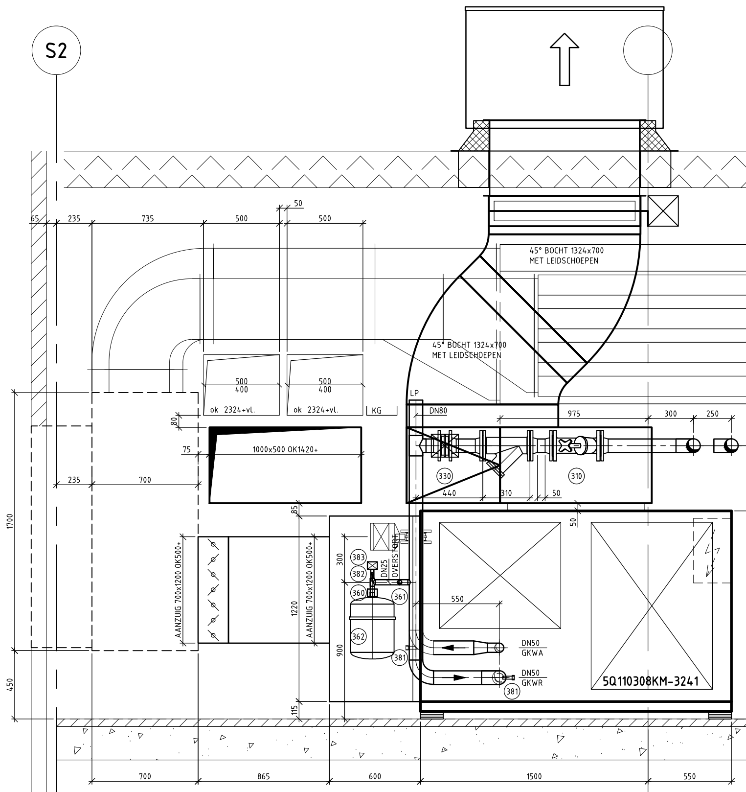
DOORSNEDE B-B
