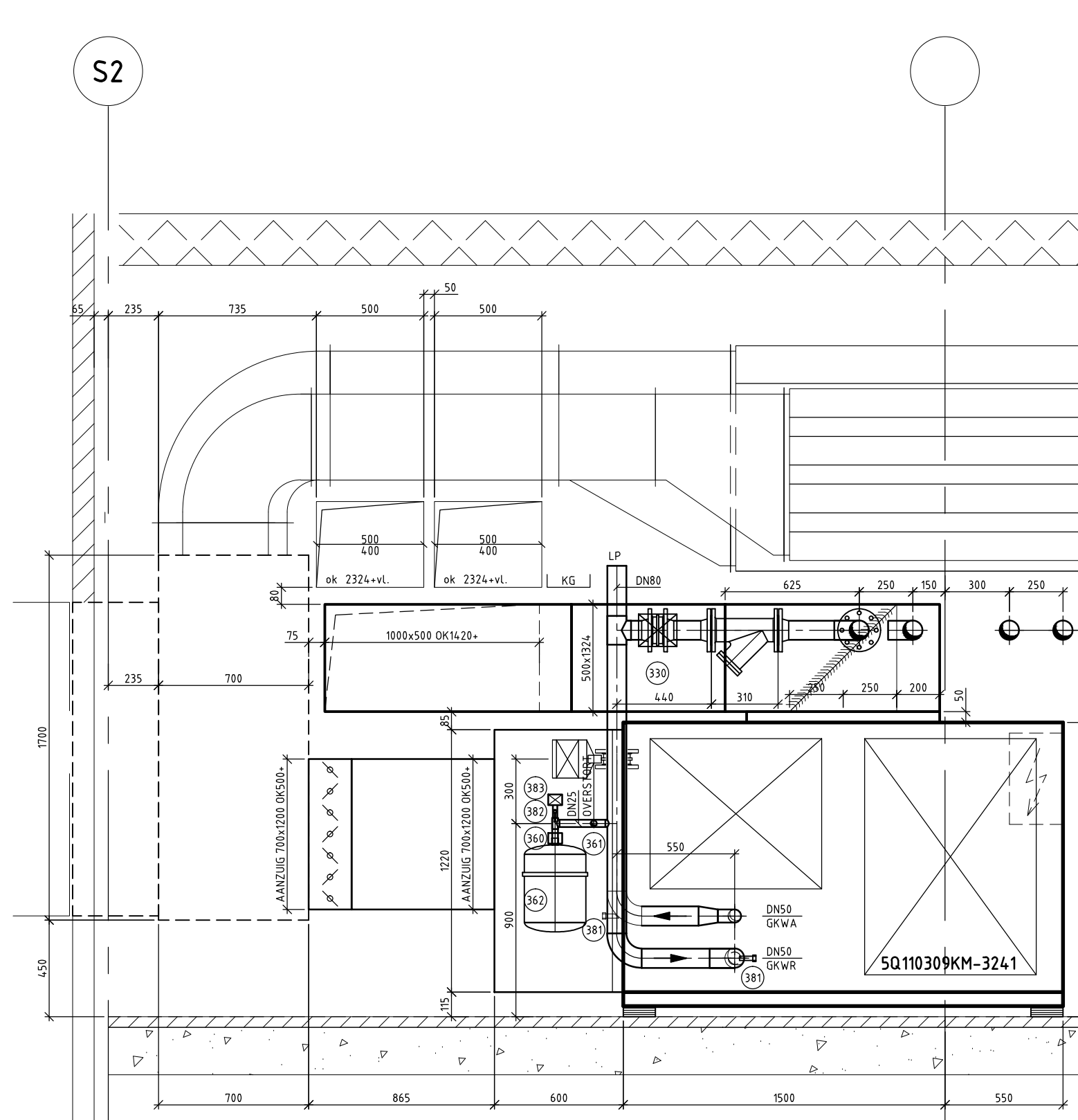
DOORSNEDE C-C
