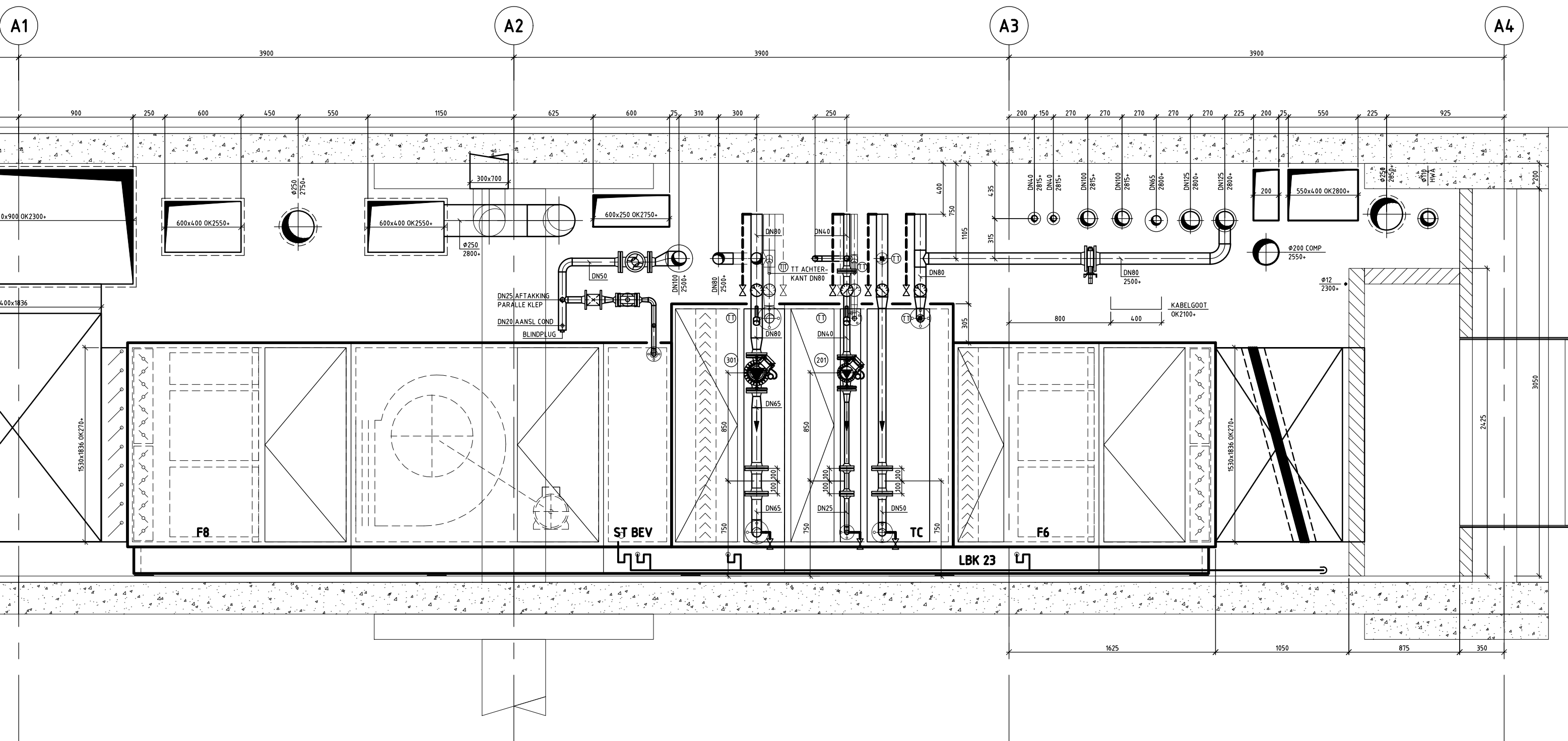
DOORSNEDE D-D SCHAAL 1:20
